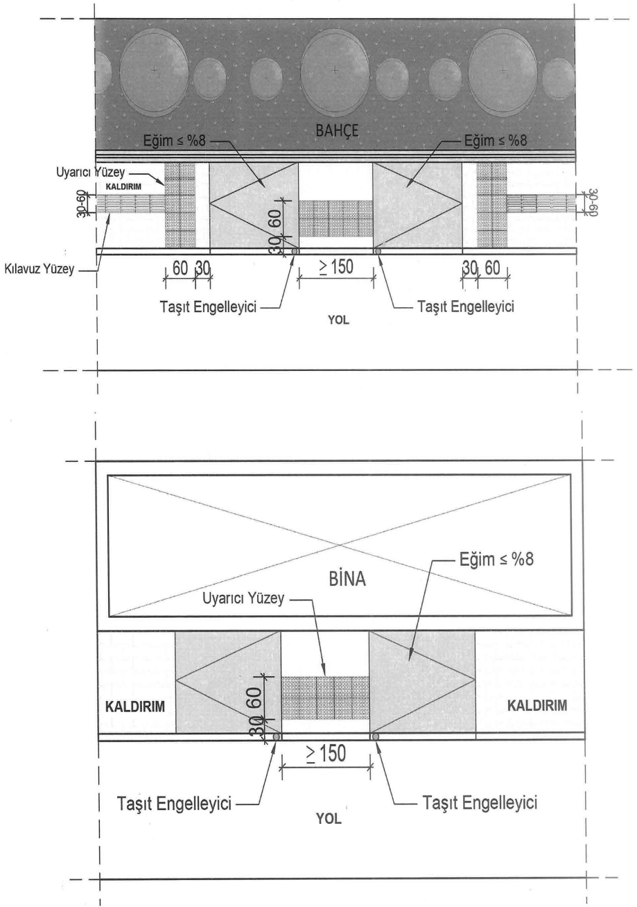
Şekil-4 Kaldırımın dar olması durumunda yola paralel kaldırım rampaları
