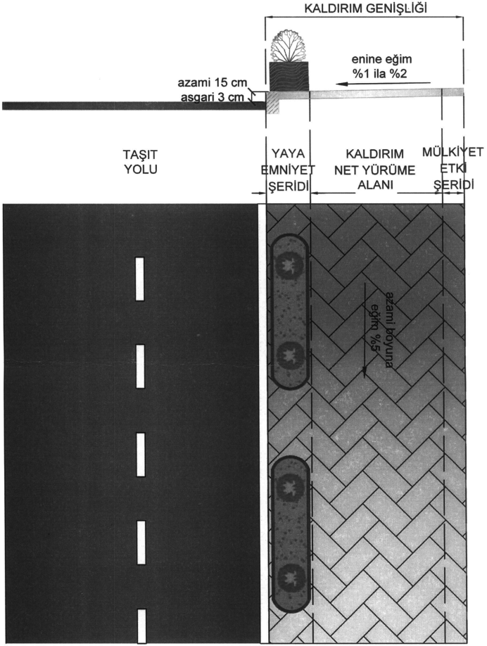
Şekil-1 Yaya emniyet şeridi, kaldırım net yürüme alanı ve mülkiyet etki şeridi gösterimi
