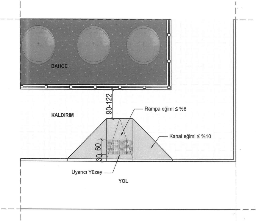
Şekil-2 Üç yöne eğimli kaldırım rampaları
