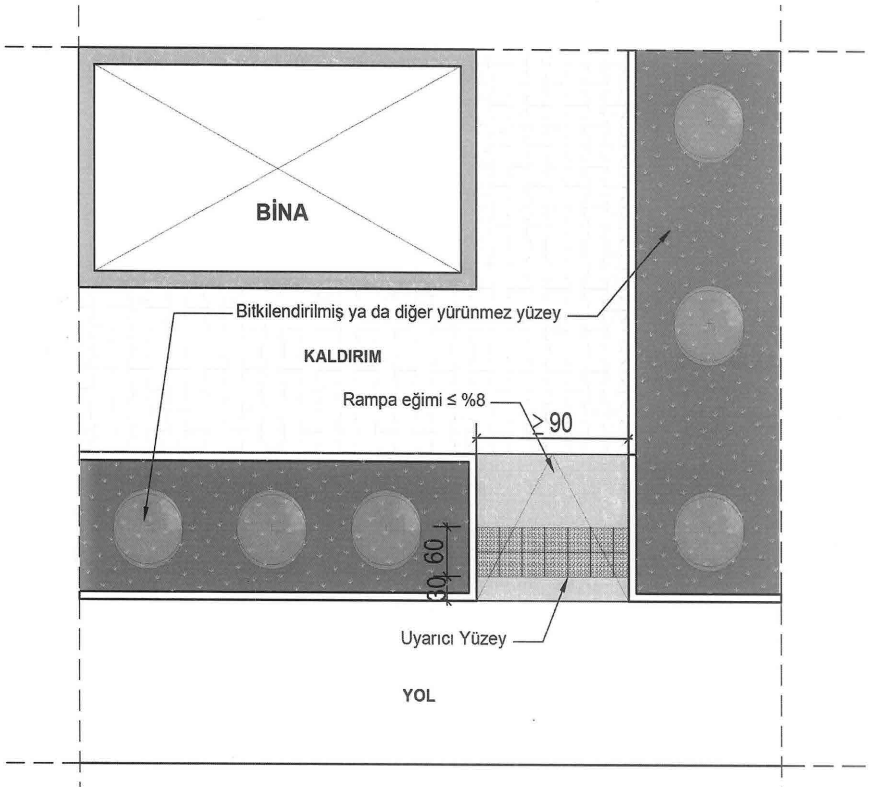
Şekil-3 Tek yöne eğimli kaldırım rampaları
